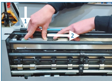
EasyBlade-Schnellverschlussmechanismus
