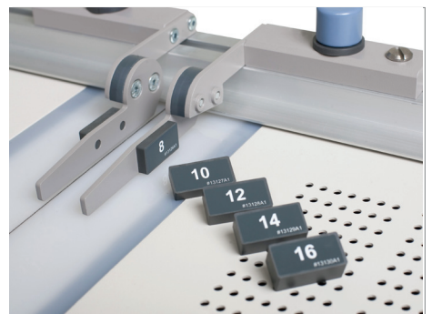
Auswechselbare Abstandshalter (Quick-change Spacers) zum Definieren der Scharnierbreite (Abstand zwischen Rückensteg und Decke)
