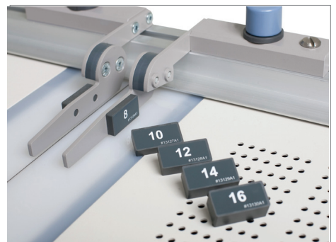
Auswechselbare Abstandshalter (Quick-change Spacers) zum Definieren der Scharnierbreite (Abstand zwischen Rückensteg und Decke)
